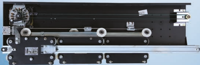
Teleskobik 3 Panel Kabin Operatörü 3 Panels Telescopic Car Door Operator Opérateur de Porte Cabine Télescopique, 3 Vantaux
